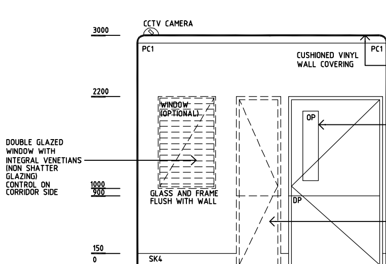
ELEVATION 1
