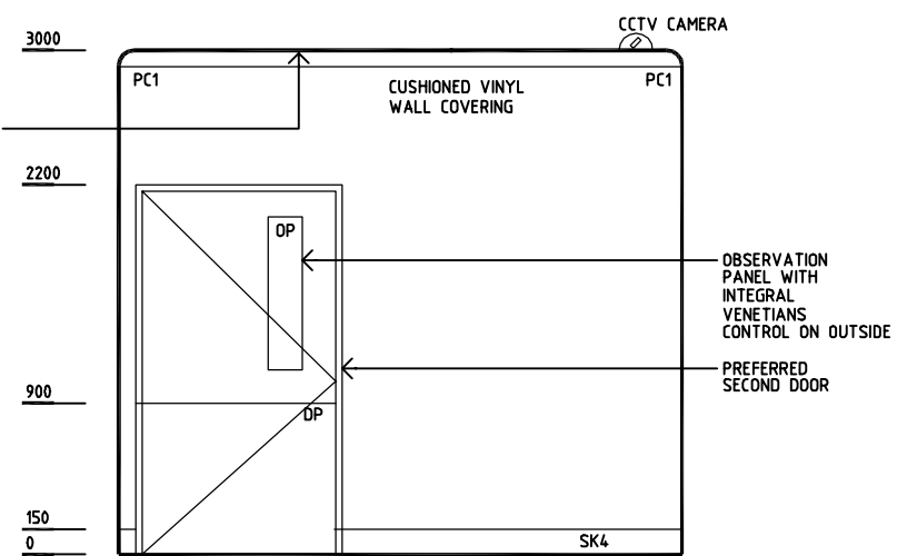
ELEVATION 2
