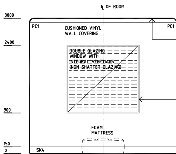
ELEVATION 1
