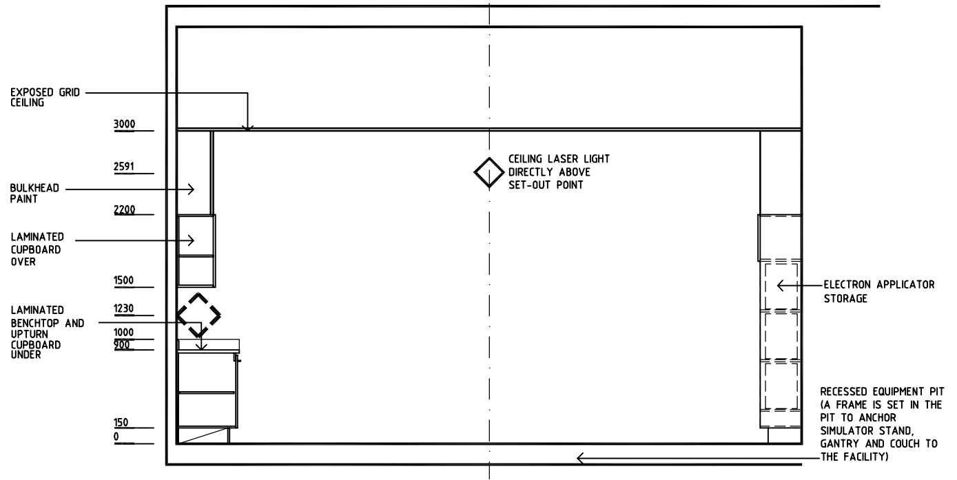
ELEVATION 2
