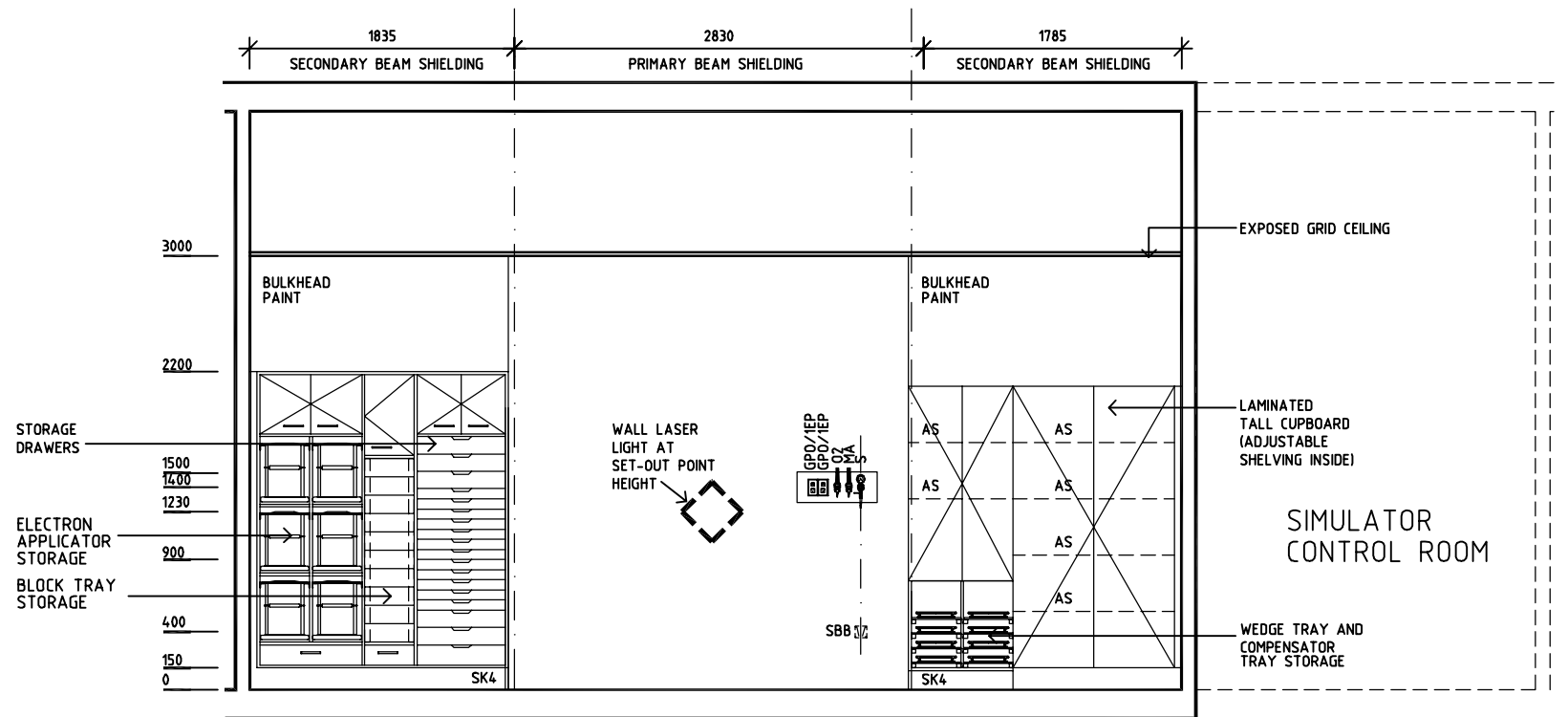
ELEVATION 3
