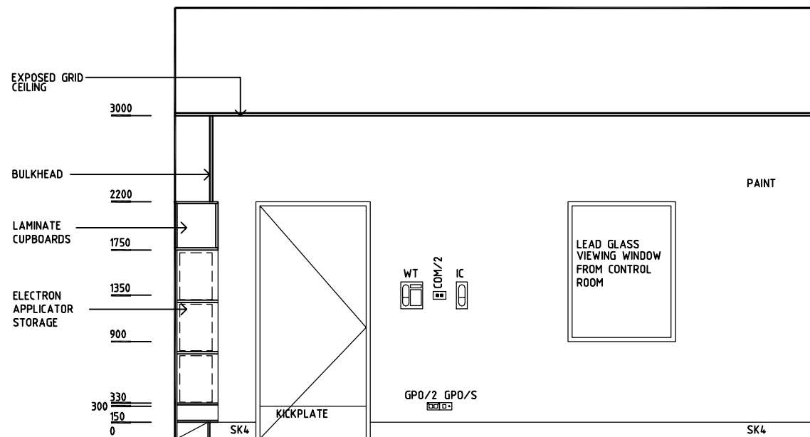
ELEVATION 4
