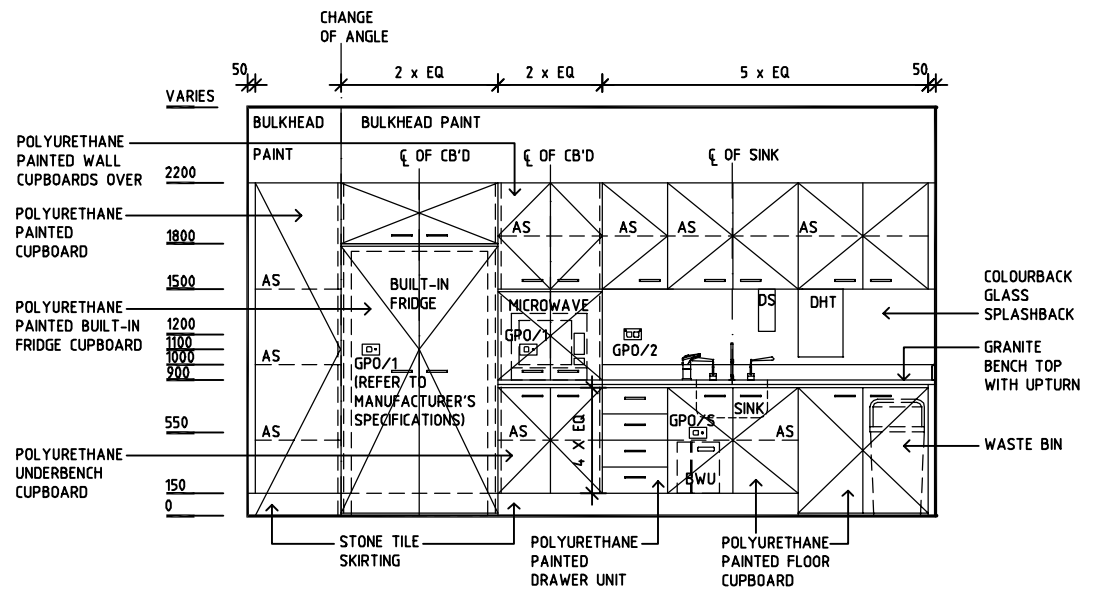
ELEVATION 2
