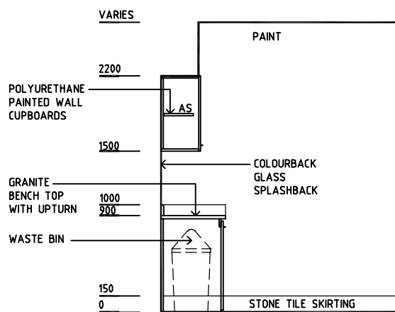
ELEVATION 3
