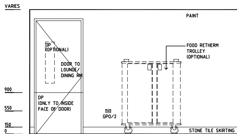
ELEVATION 4
