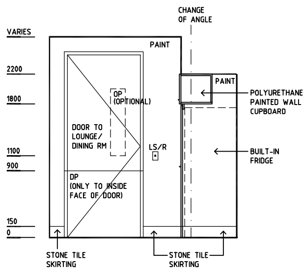
ELEVATION 1
