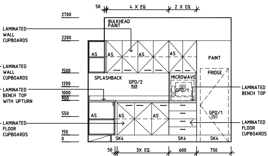
ELEVATION 2
