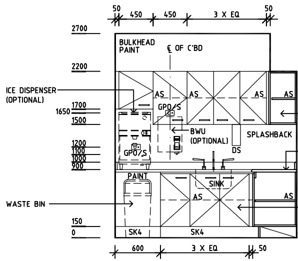
ELEVATION 1
