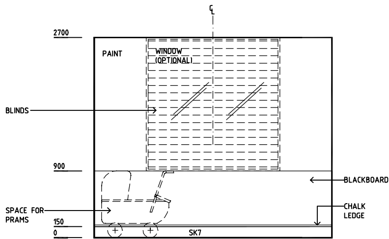
ELEVATION 1
