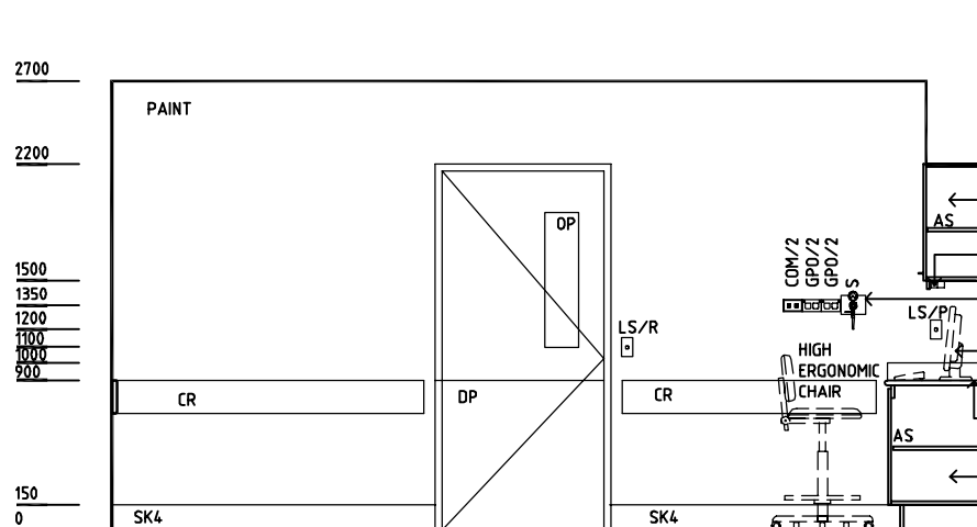
ELEVATION 1
