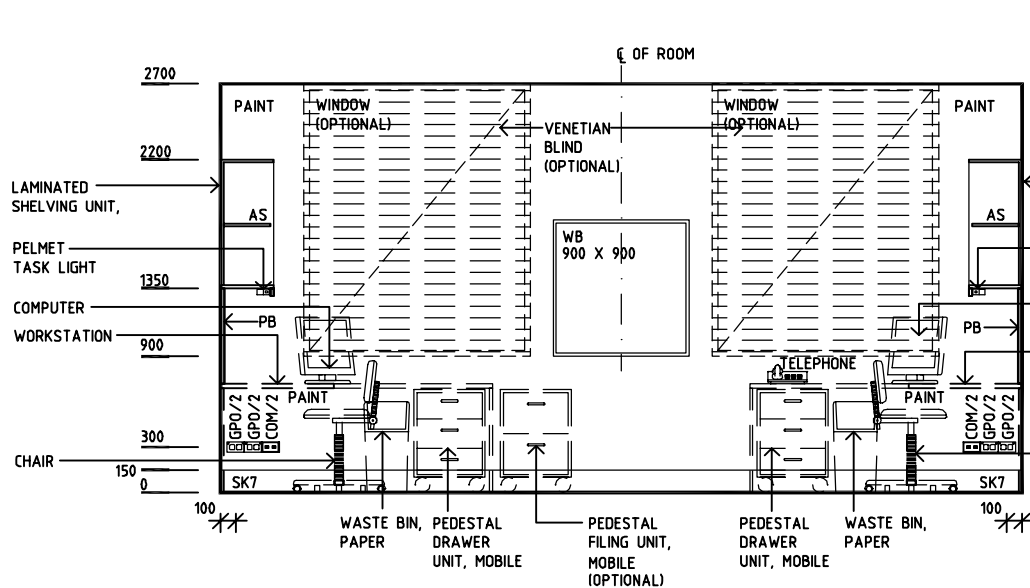
ELEVATION 1
