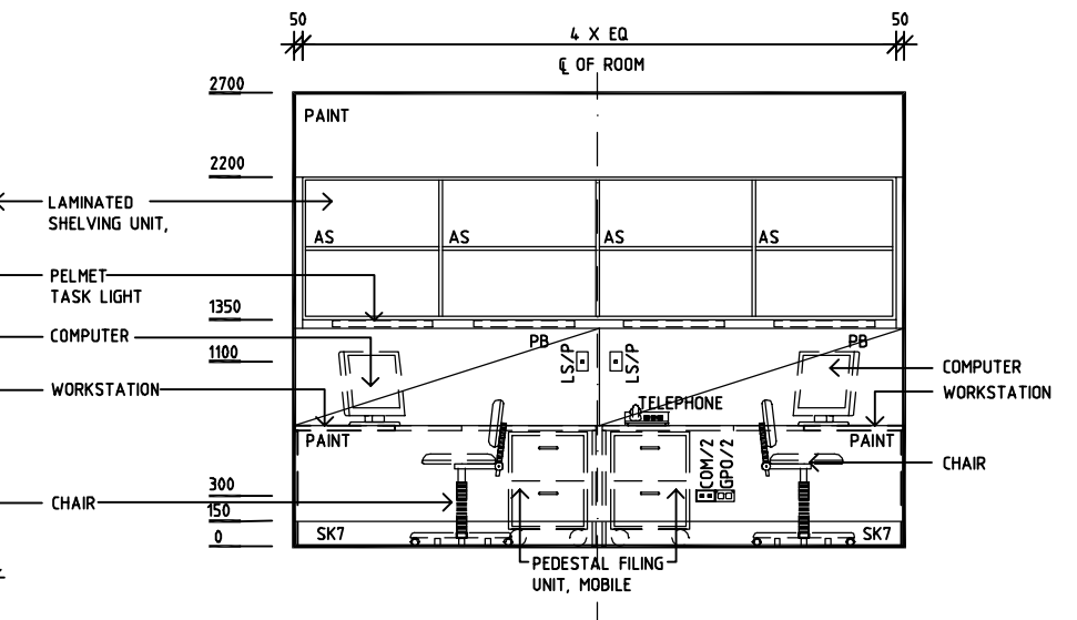
ELEVATION 2
