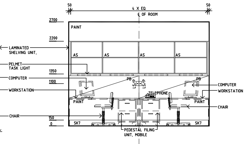
ELEVATION 4
