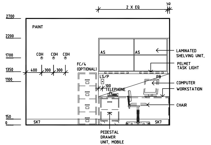
ELEVATION 4
