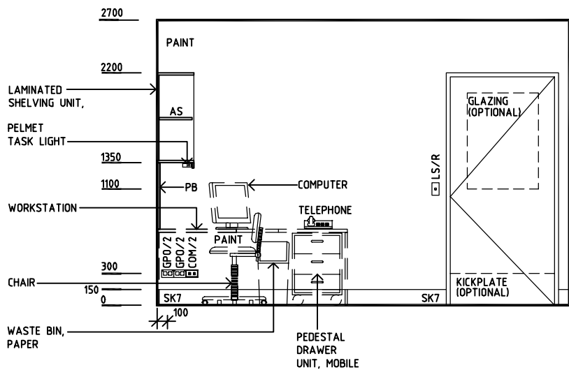
ELEVATION 3
