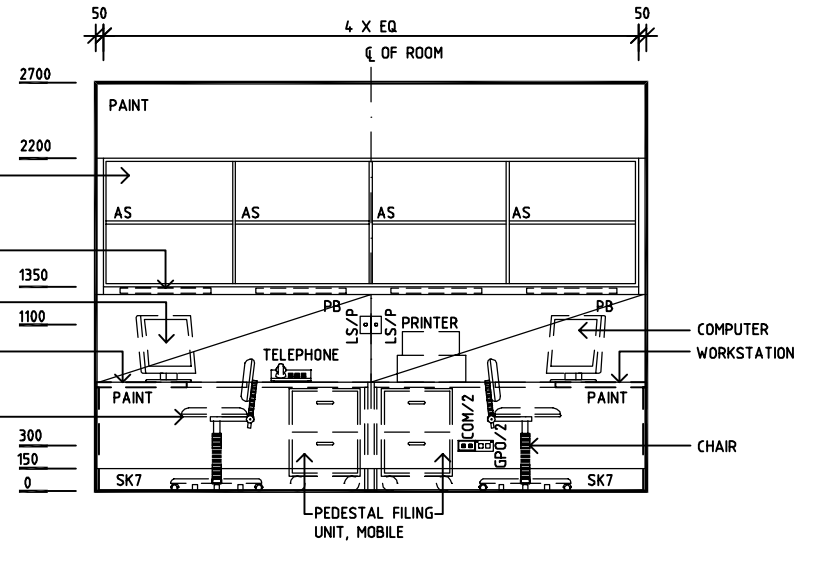
ELEVATION 2
