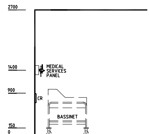
ELEVATION 2
