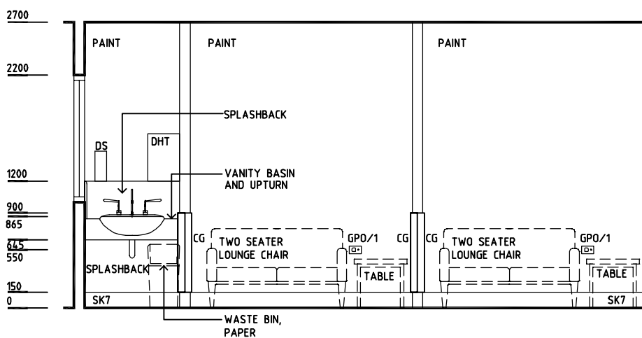
ELEVATION 3
