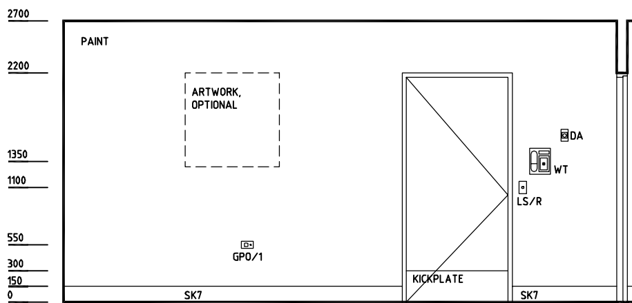
ELEVATION 1
