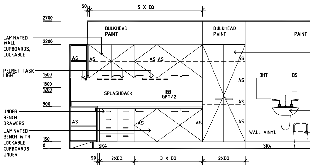
ELEVATION 1
