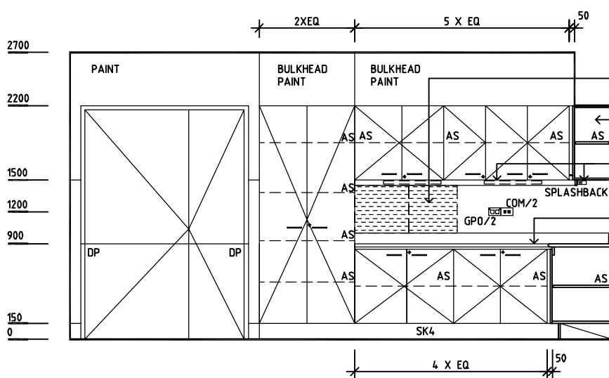
ELEVATION 3
