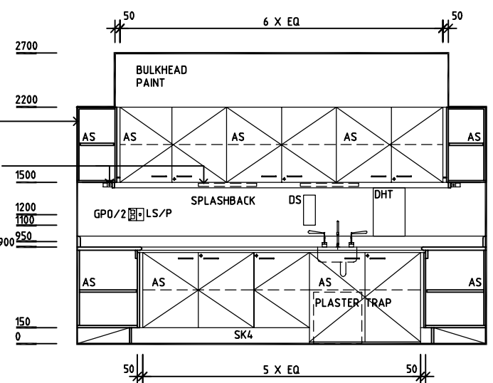
ELEVATION 4
