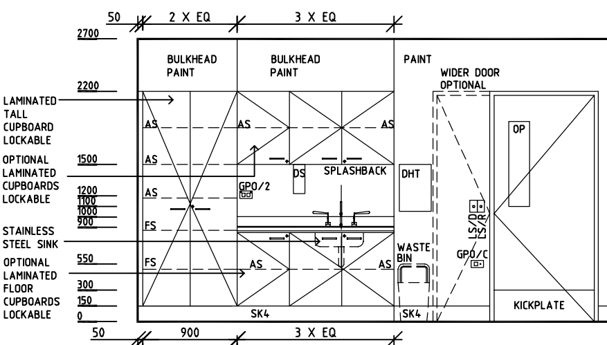
ELEVATION 3
