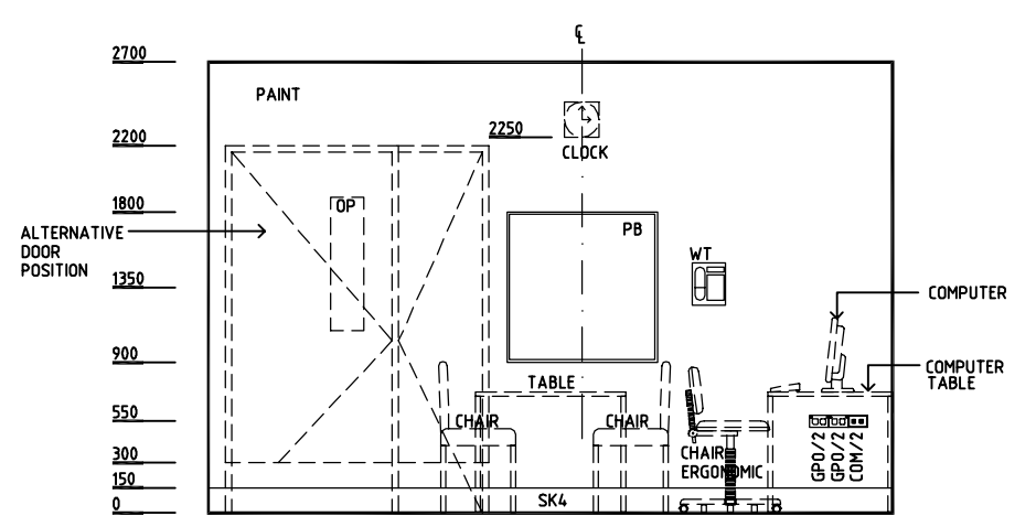
ELEVATION 4
