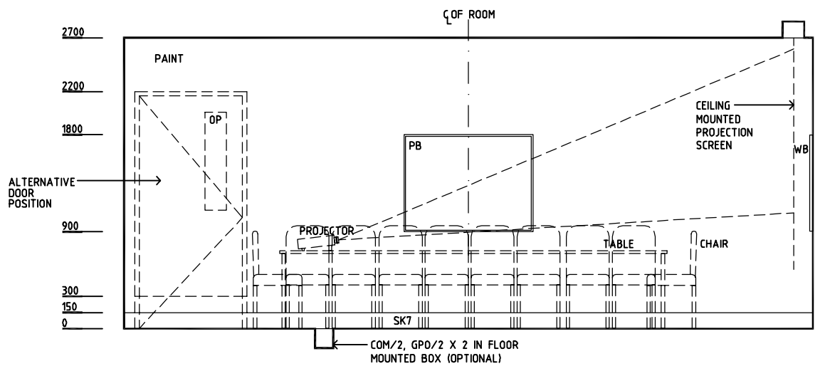
ELEVATION 4
