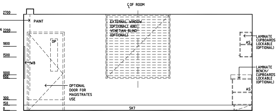
ELEVATION 2
