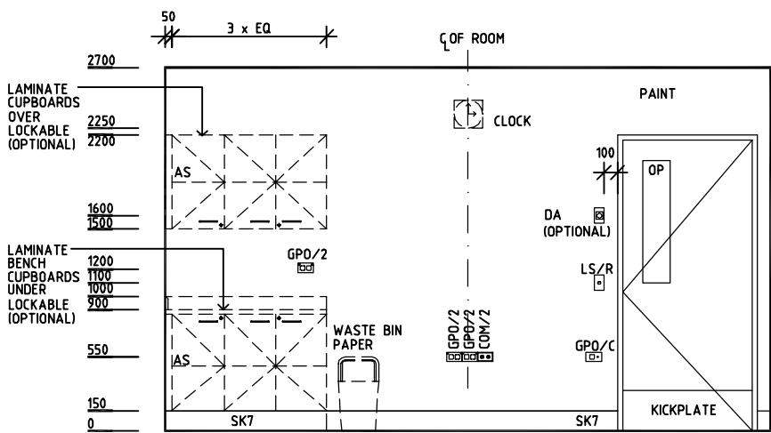
ELEVATION 1
