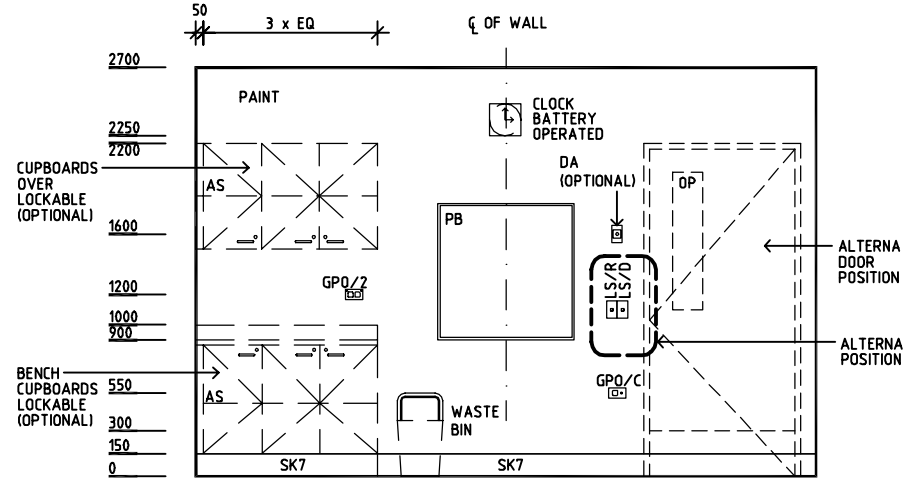
ELEVATION 2
