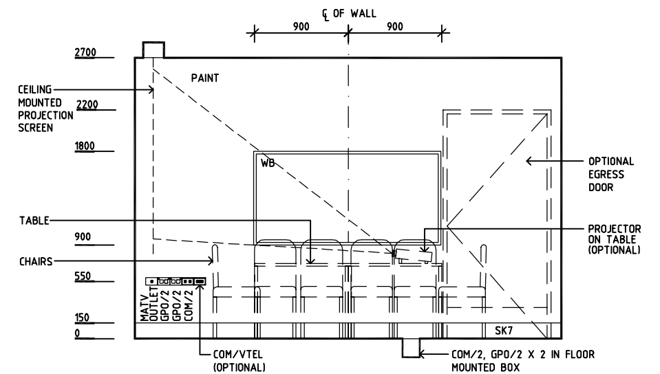
ELEVATION 4
