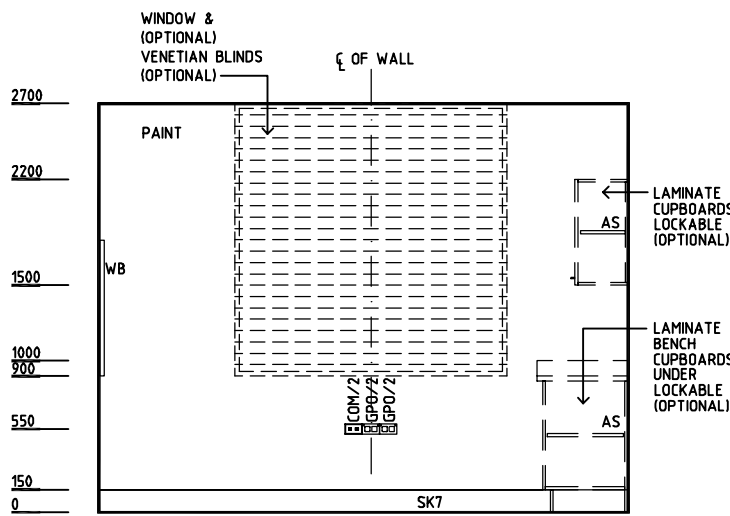
ELEVATION 1
