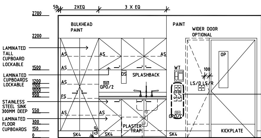
ELEVATION 3
