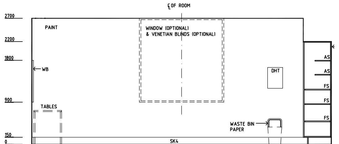
ELEVATION 2
