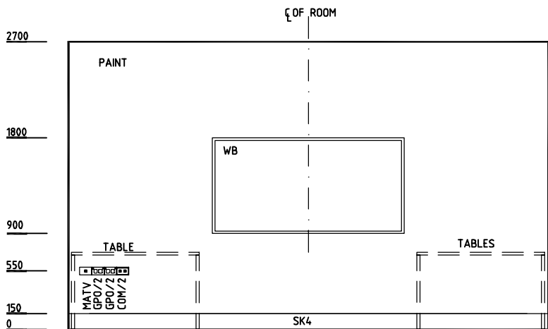
ELEVATION 1
