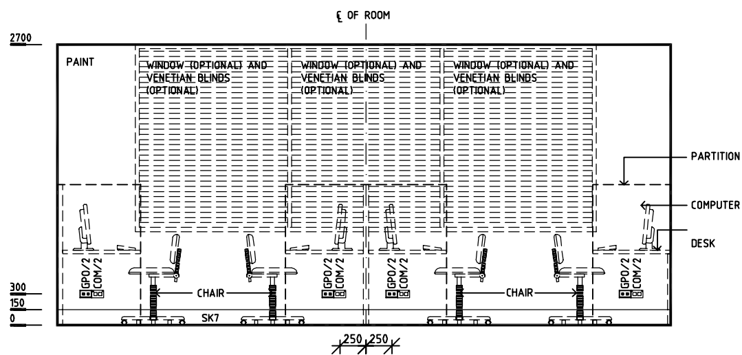
ELEVATION 1
