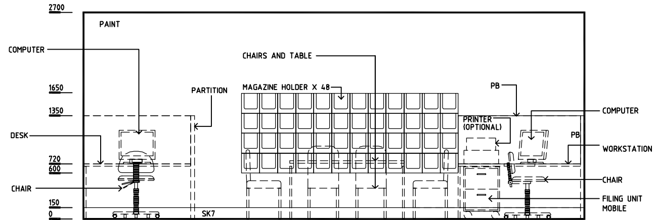
ELEVATION 2
