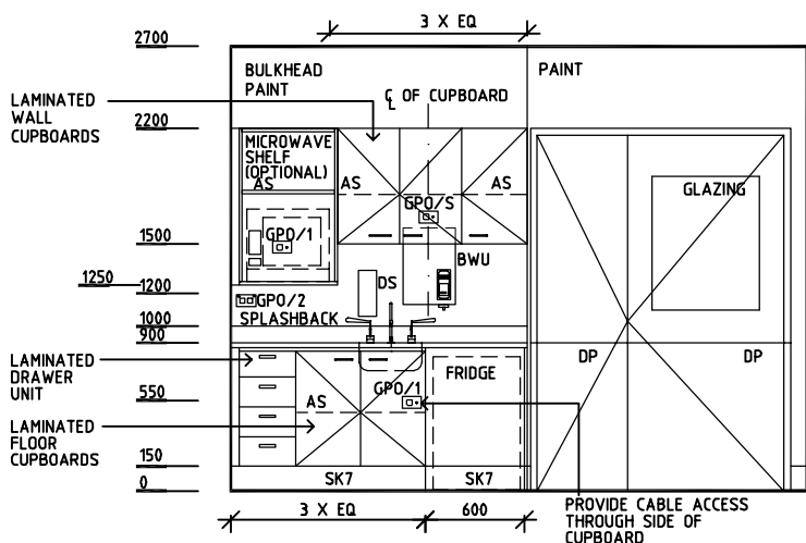
ELEVATION 3
