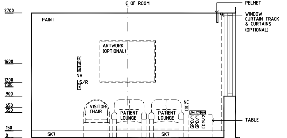
ELEVATION 2
