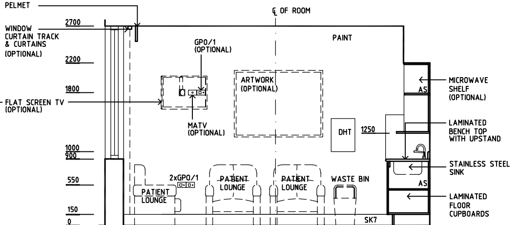
ELEVATION 2
