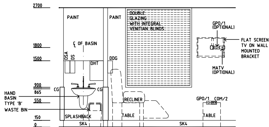
ELEVATION 2
