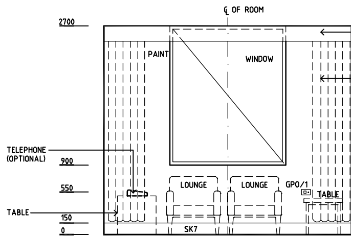
ELEVATION 1
