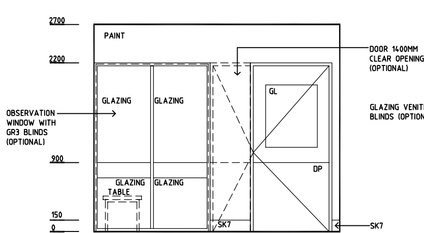
ELEVATION 3
