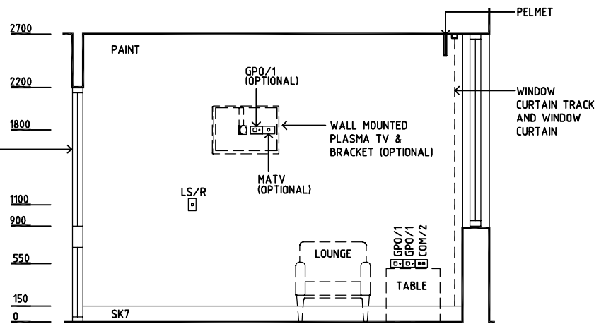
ELEVATION 4
