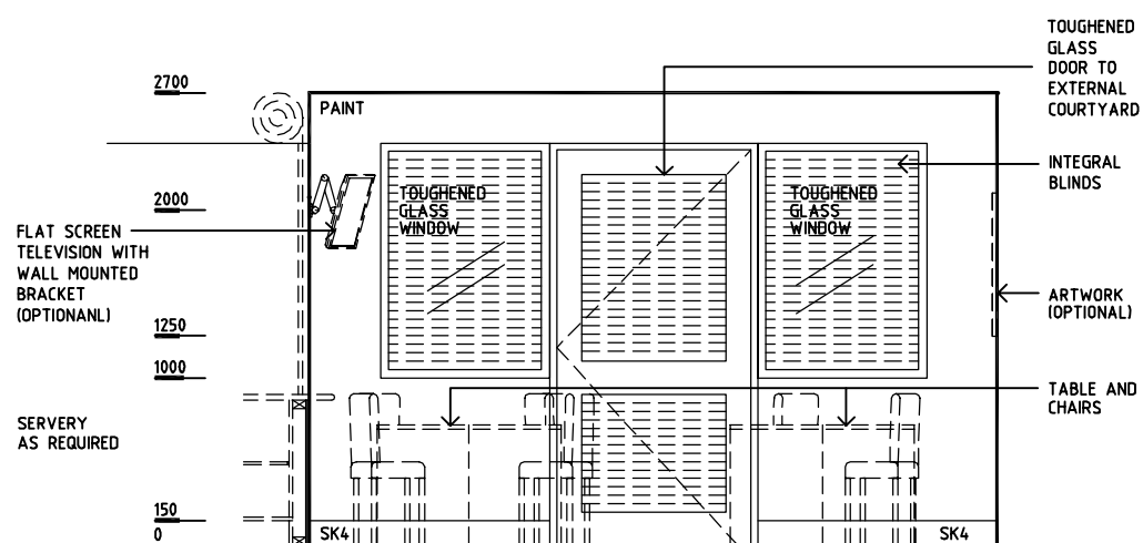
ELEVATION 1
