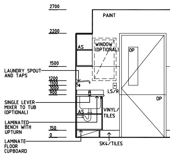
ELEVATION 3
