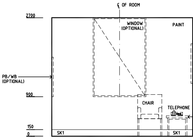
ELEVATION 1
