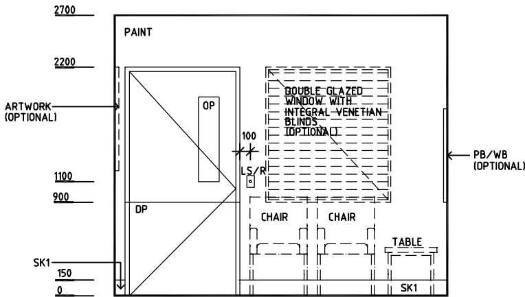
ELEVATION 3
