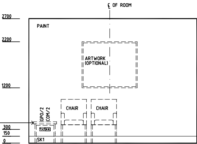
ELEVATION 2
