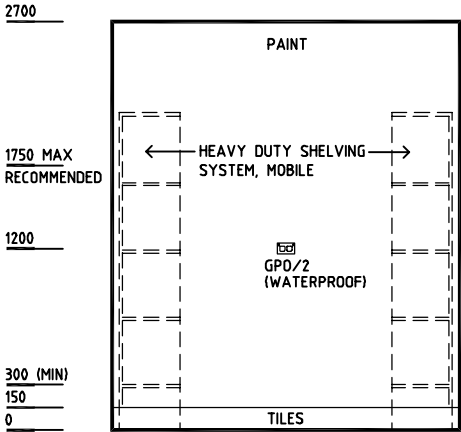
ELEVATION 2
