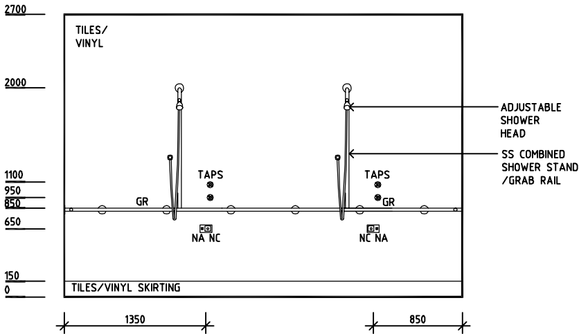
ELEVATION 3
