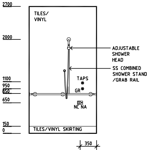
ELEVATION 4
