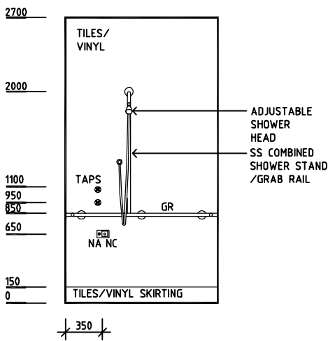
ELEVATION 2
