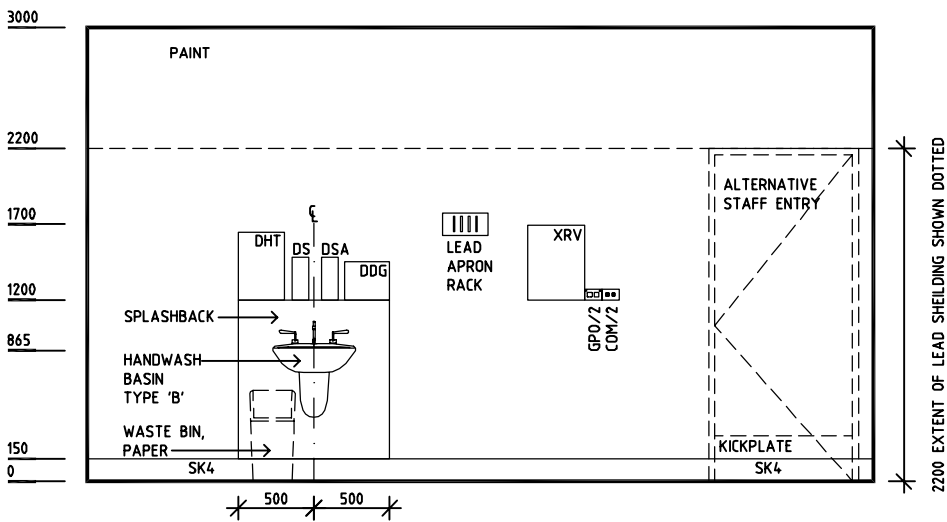
ELEVATION 4
