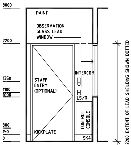
ELEVATION 6
