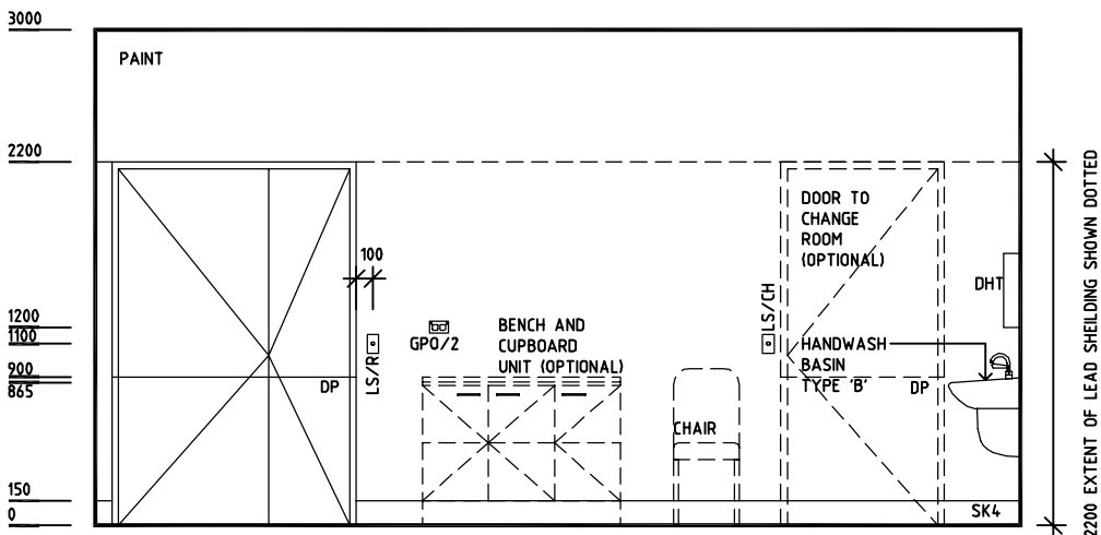
ELEVATION 3
