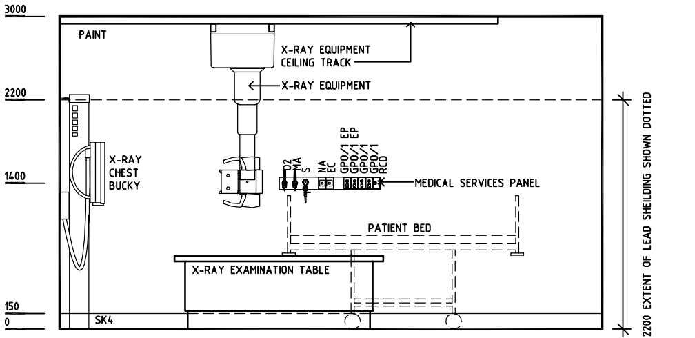
ELEVATION 2
