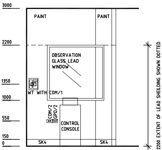
ELEVATION 5
