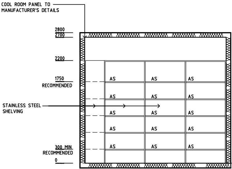
ELEVATION 1
