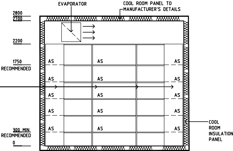
ELEVATION 4
