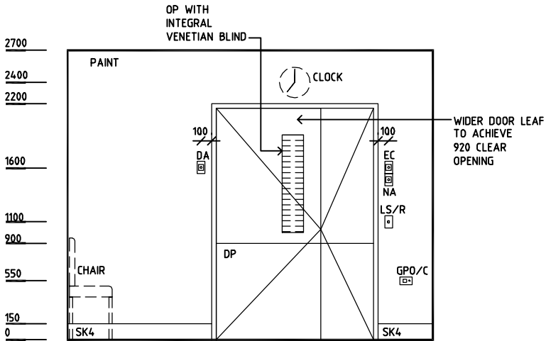
ELEVATION 3
