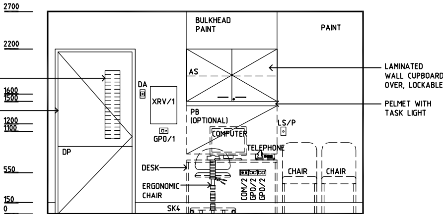
ELEVATION 2
