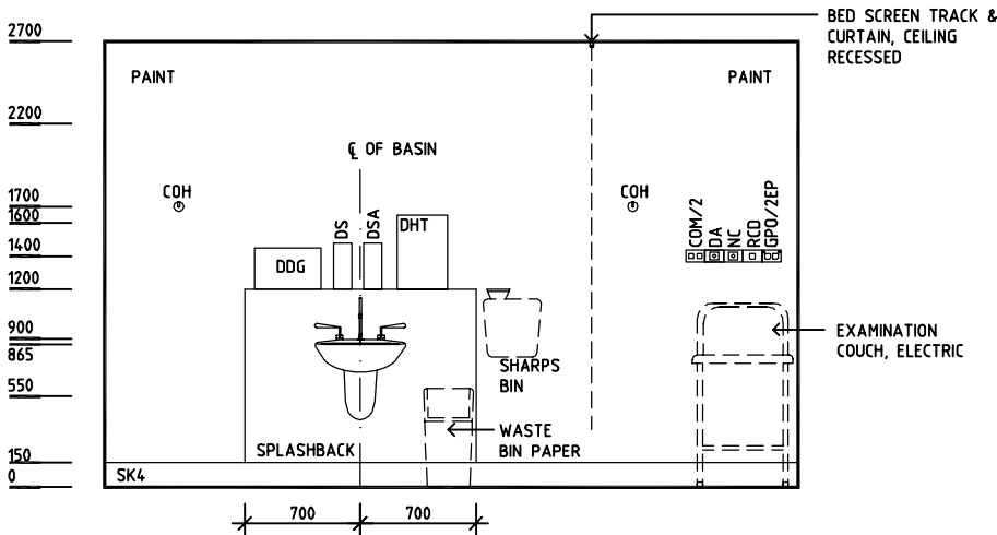
ELEVATION 4
