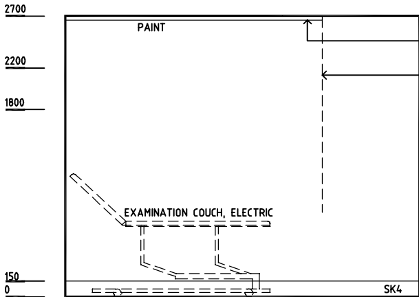
ELEVATION 1
