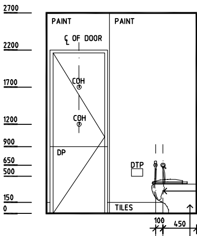
ELEVATION 1
