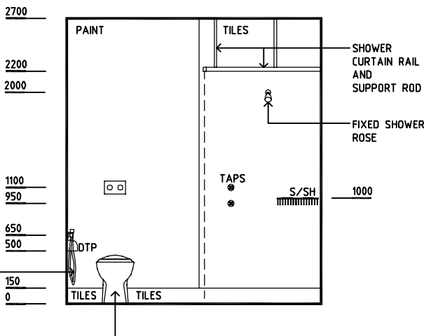
ELEVATION 2
