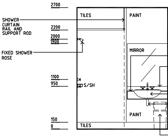
ELEVATION 3
