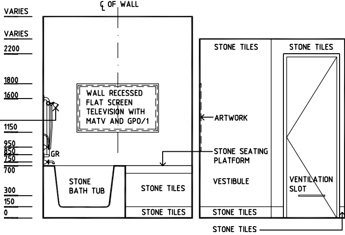
ELEVATION 4
