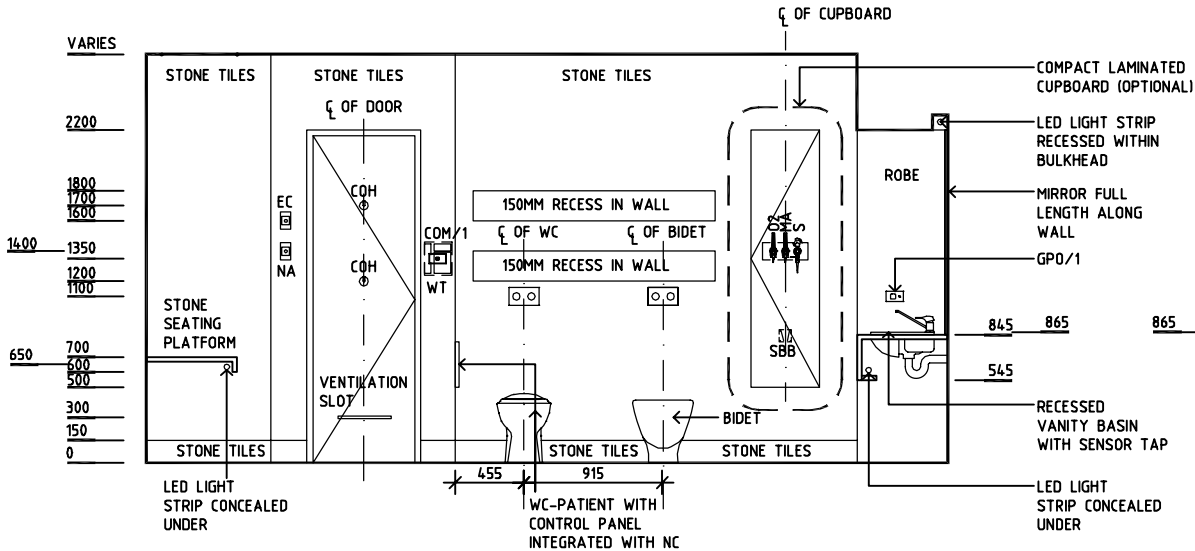
ELEVATION 1
