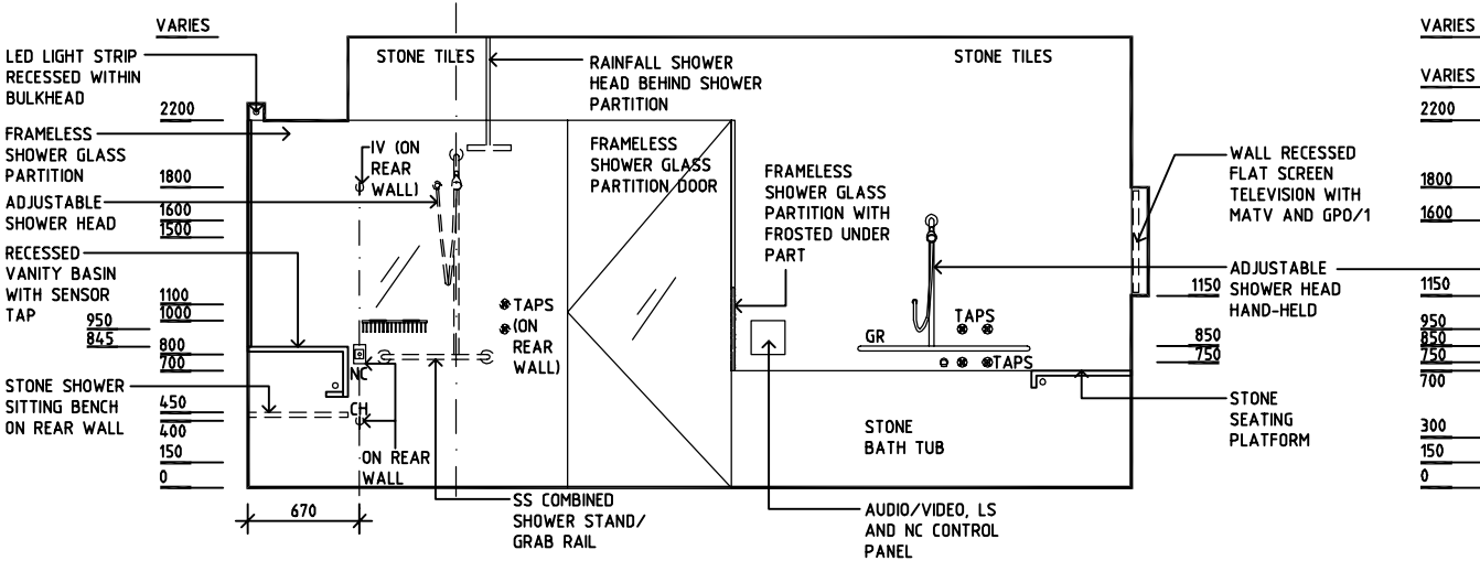
ELEVATION 3
