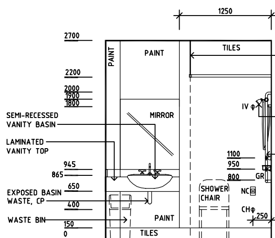
ELEVATION 1
