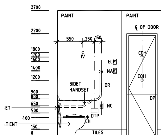
ELEVATION 3
