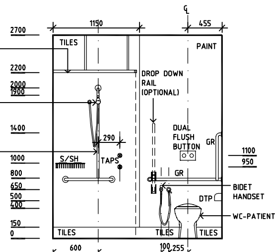
ELEVATION 2
