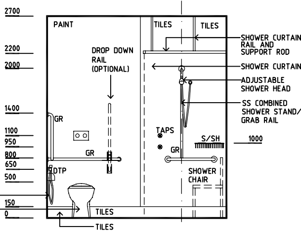
ELEVATION 2
