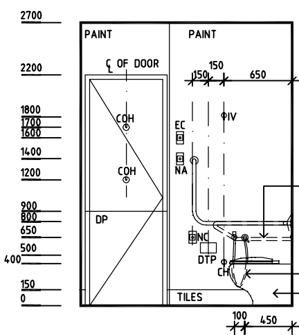
ELEVATION 1
