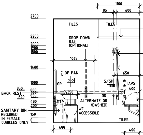
ELEVATION 1
