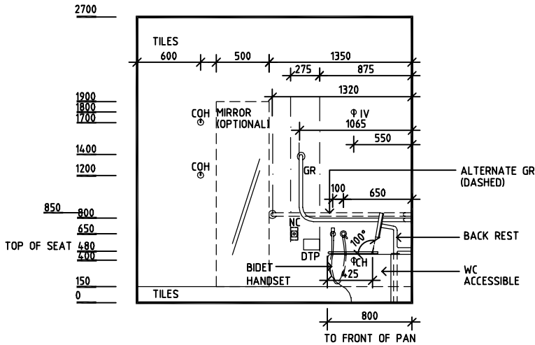
ELEVATION 4
