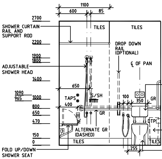
ELEVATION 3
