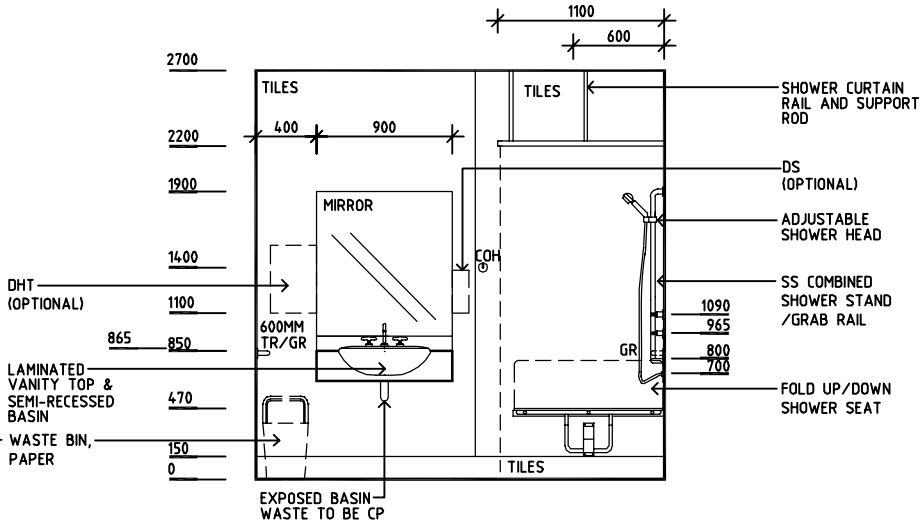
ELEVATION 2
