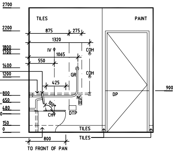
ELEVATION 4
