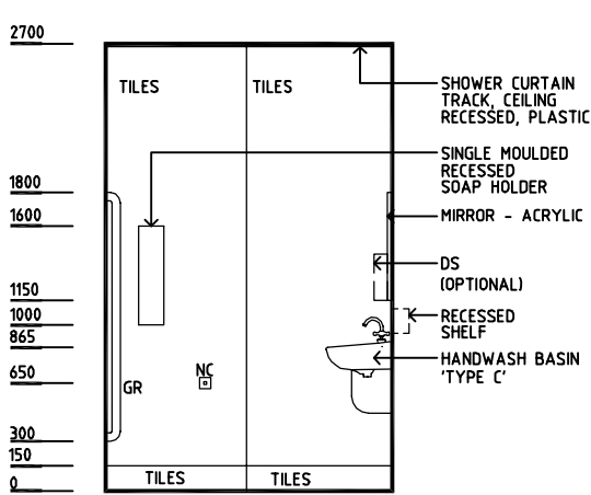
ELEVATION 4
