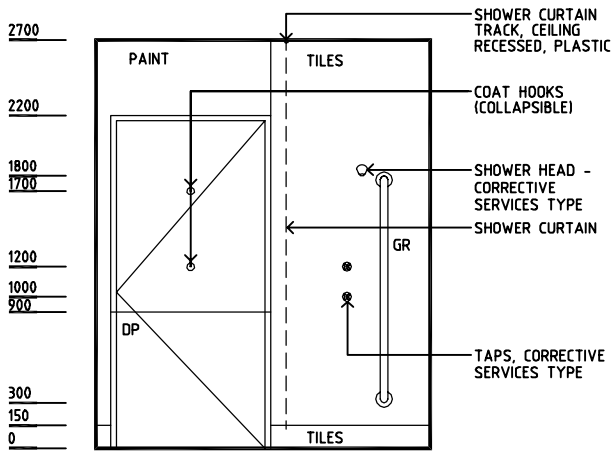
ELEVATION 3
