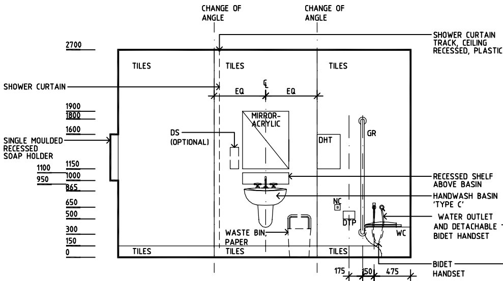
ELEVATION 1
