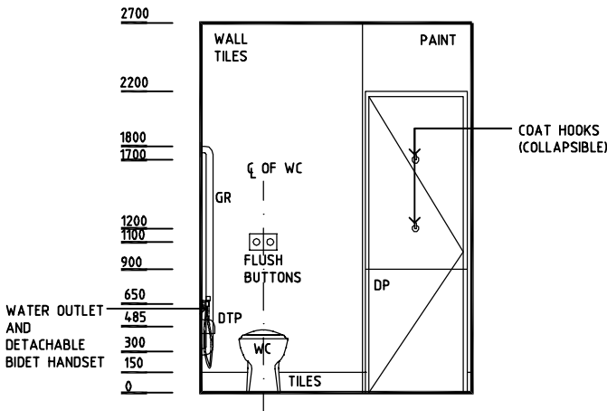
ELEVATION 4
