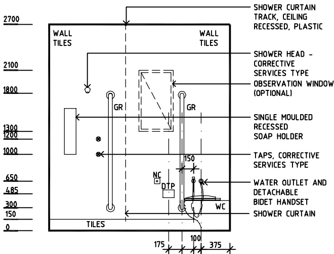
ELEVATION 3
