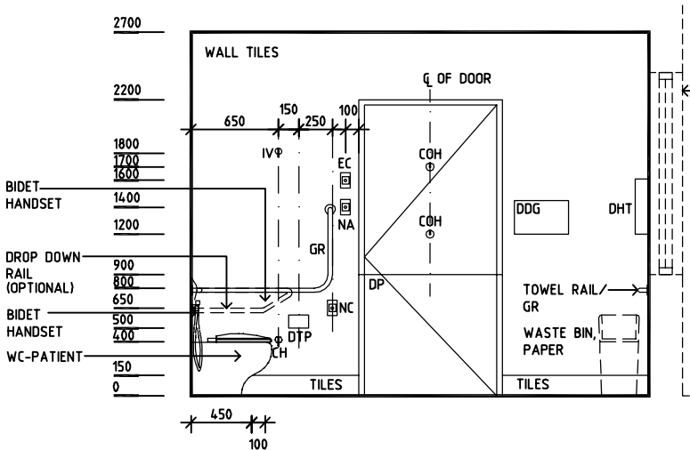
ELEVATION 1
