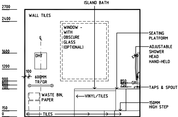
ELEVATION 2
