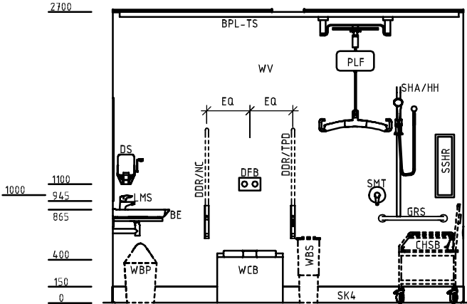
ELEVATION 4
