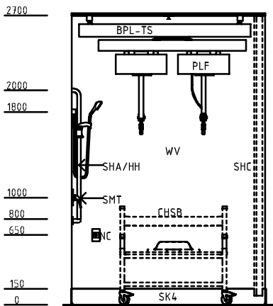
ELEVATION 1
