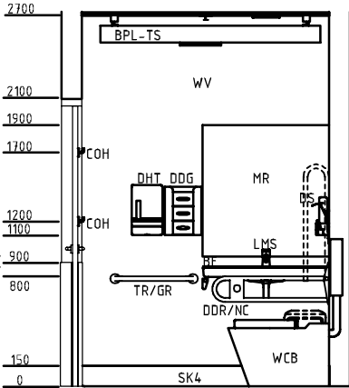
ELEVATION 3
