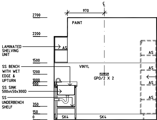
ELEVATION 1
