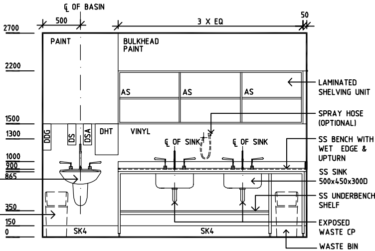
ELEVATION 4
