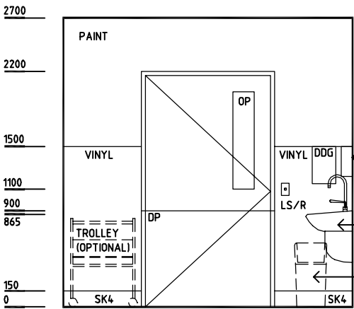
ELEVATION 3
