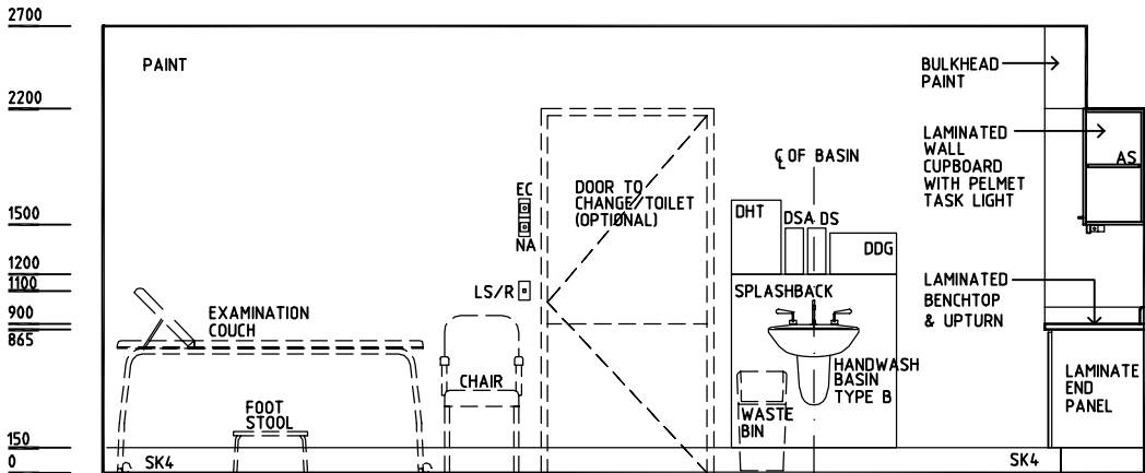
ELEVATION 2
