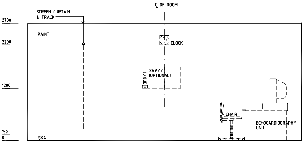
ELEVATION 4
