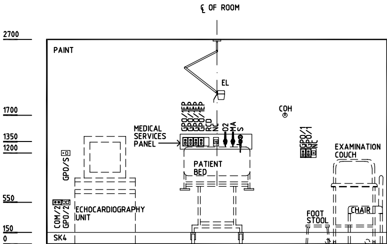
ELEVATION 1
