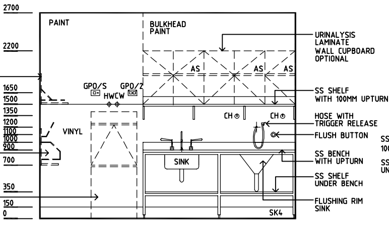
ELEVATION 2
