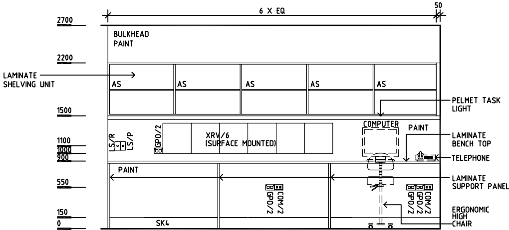
ELEVATION 3
