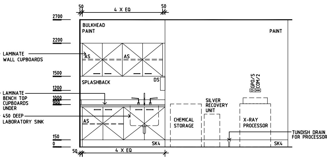
ELEVATION 2
