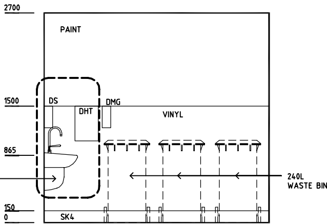
ELEVATION 4
