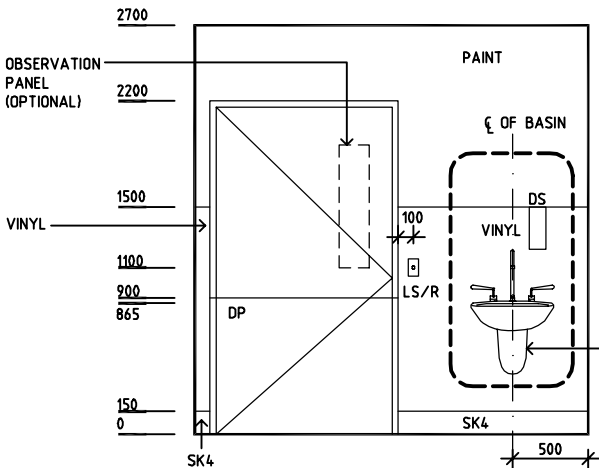
ELEVATION 3
