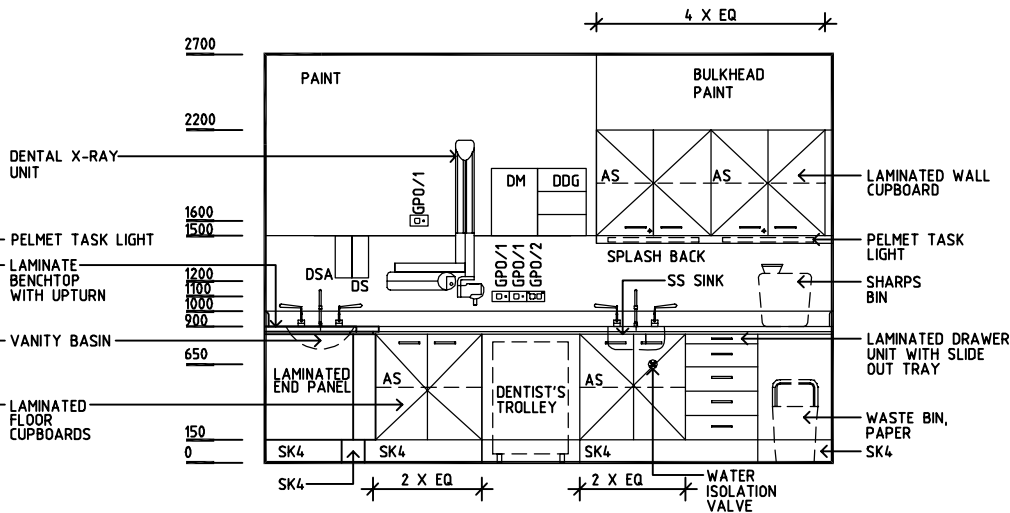
ELEVATION 4
