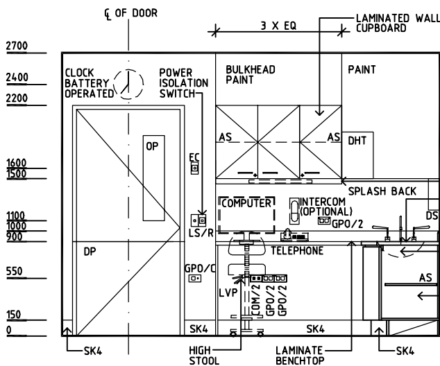
ELEVATION 3
