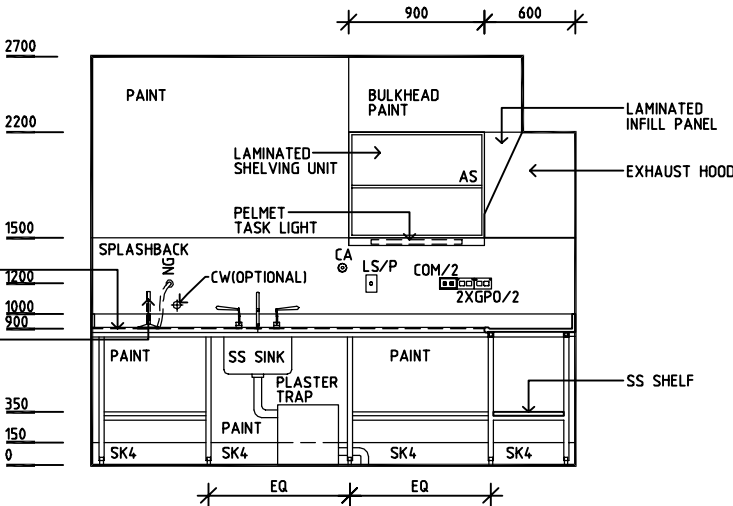
ELEVATION 4
