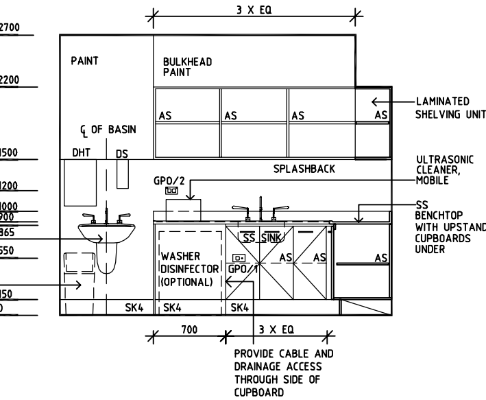
ELEVATION 4
