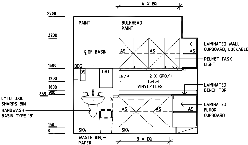
ELEVATION 4
