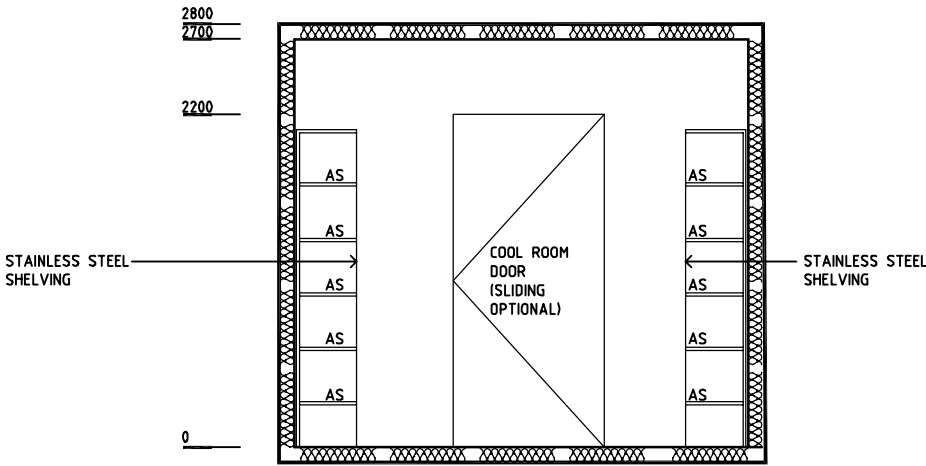
ELEVATION 2
