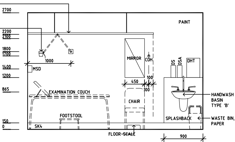
ELEVATION 2
