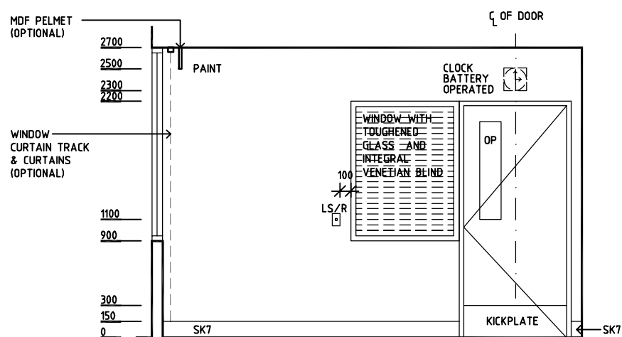
ELEVATION 3
