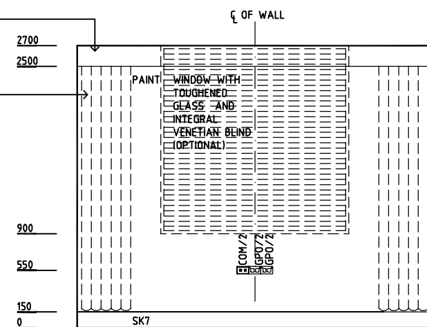
ELEVATION 2
