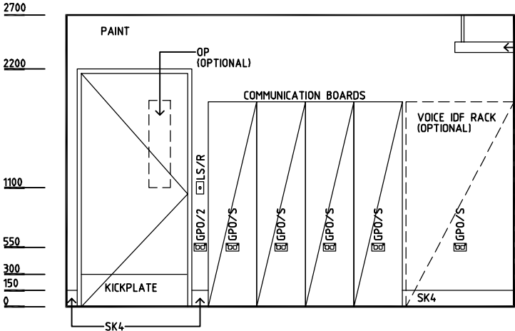
ELEVATION 3
