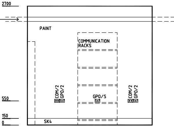
ELEVATION 4
