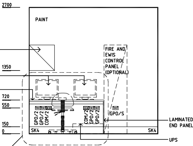
ELEVATION 2
